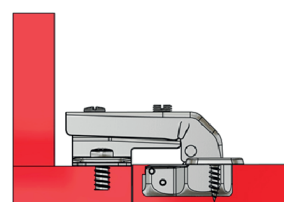
drzwi zamknięte / door close
