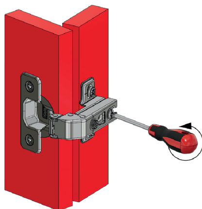
Regulacja głębi / Depth adjustment
