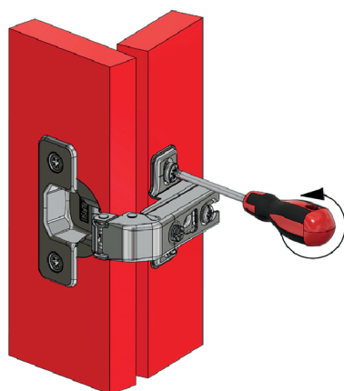
Regulacja wysokości / Height adjustment
