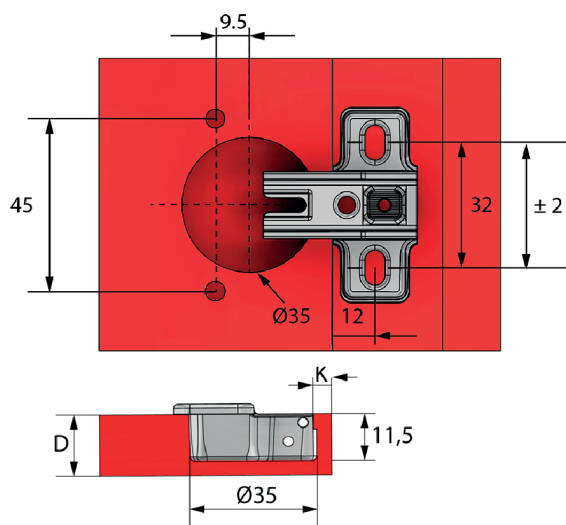
Wymiary montażowe puszki i prowadnika Drilling dimensions for the hinge cup and mounting plate
