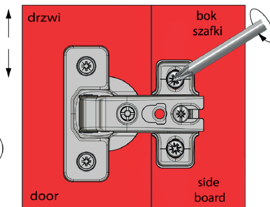
Regulacja wysokości / Height adjustment
