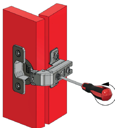
Regulacja boczna / Side adjustment
