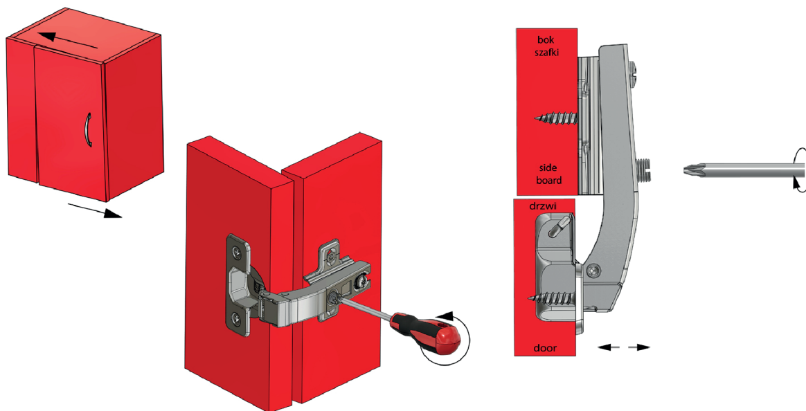
Regulacja boczna / Side adjustment
