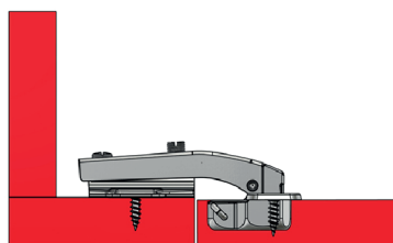
drzwi zamknięte / door close
