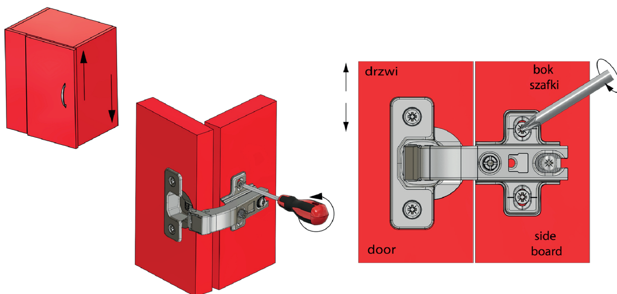
Regulacja wysokości / Height adjustment
