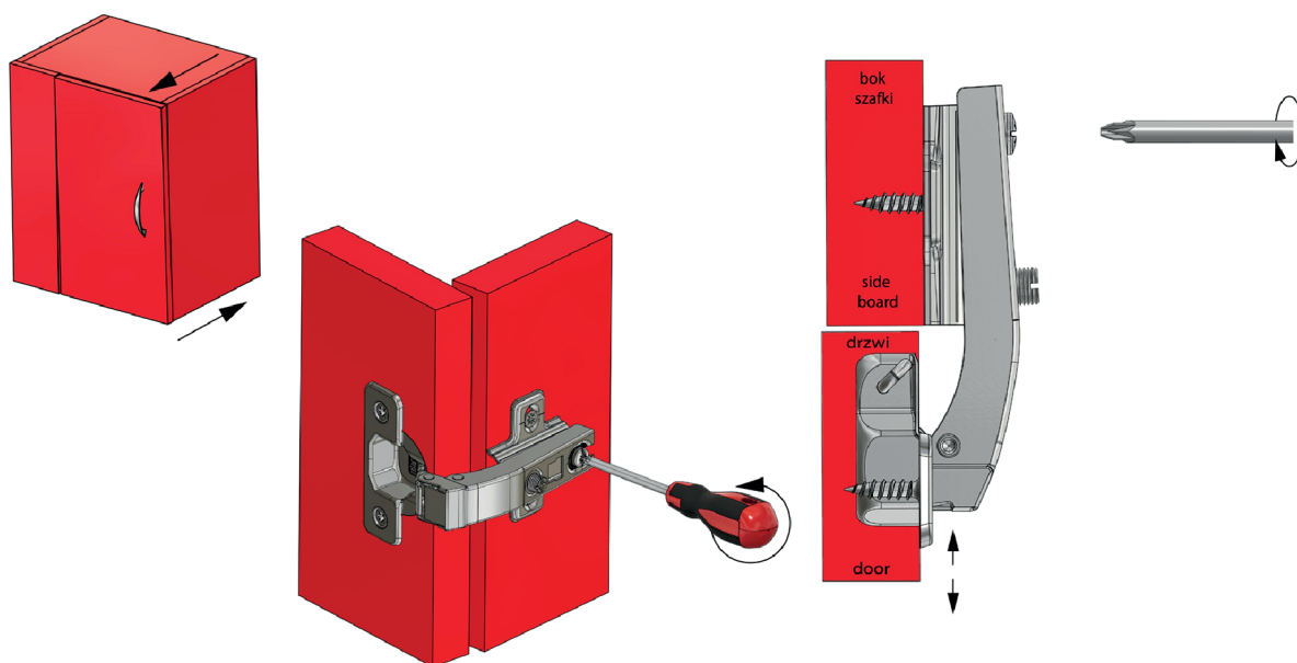
Regulacja głębi / Depth adjustment
