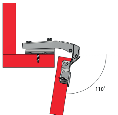
drzwi otwarte / door open
