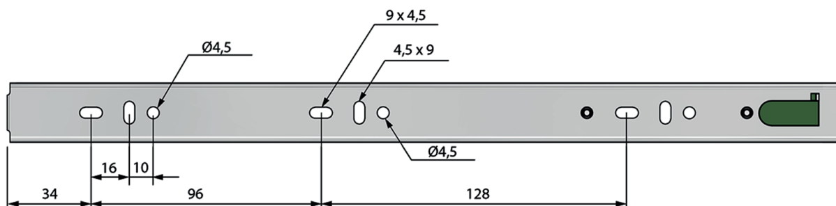
Wymiary montażowe prowadnicy szuflady Mounting dimensions for drawer slide
